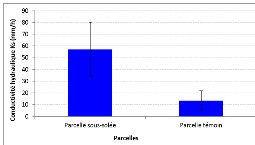
Figure 4 : Valeurs de conductivité hydraulique mesurées sur la parcelle sous-solée et son témoin.
