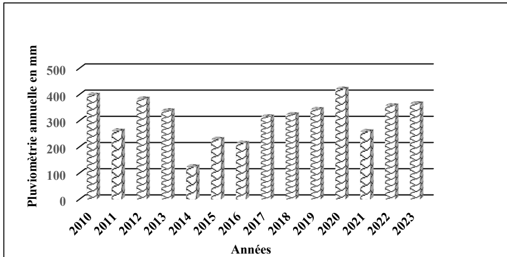
Figure 2 : Variation de la pluviométrie annuelle de la région de Saint-Louis de 2010 à 2023
