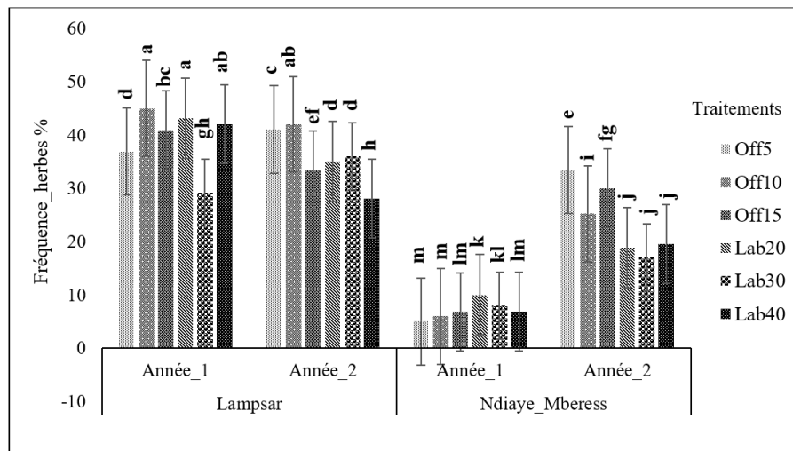
Figure 6 : Fréquence spécifique moyenne des adventices en fonction des traitements
