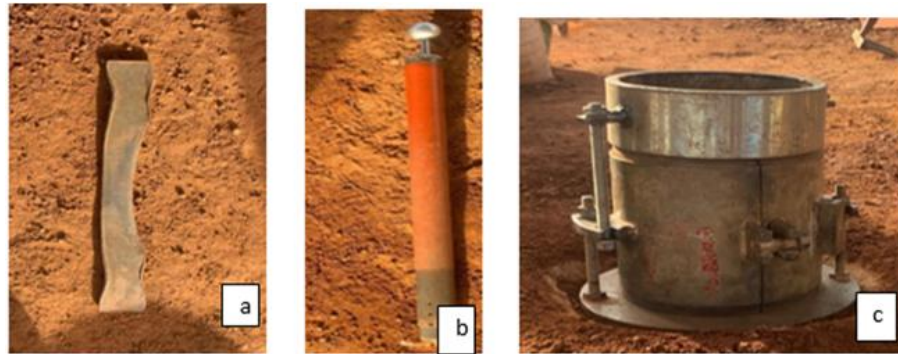
Figure 4 : Matériel essentiel pour l'essai Proctor (a-Lame à raser ; b- Dame Proctor modifiée ; c- Moule Proctor)
